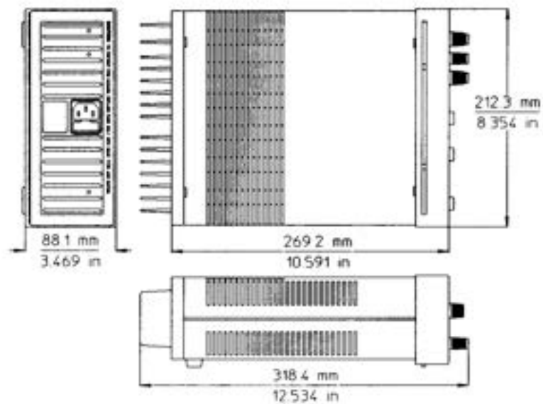
圖 1 輪廓圖解
