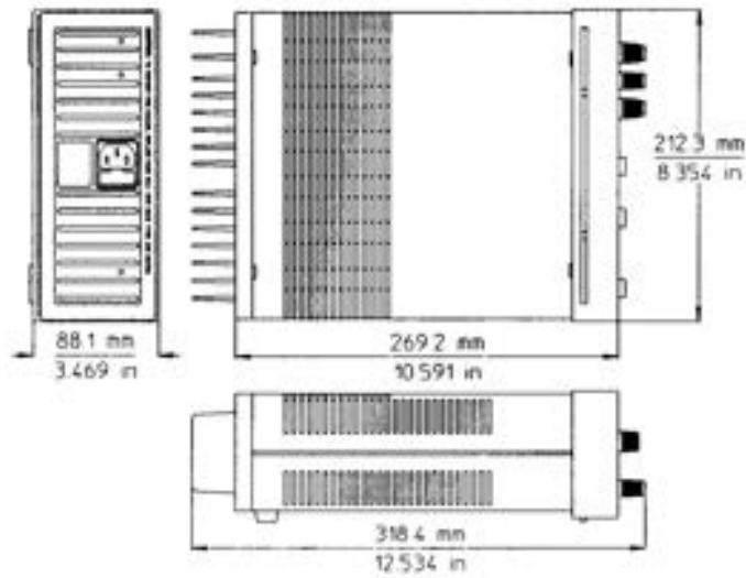
그림 1: 외형도
