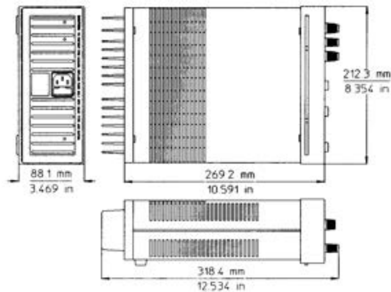
图 1 轮廓图
