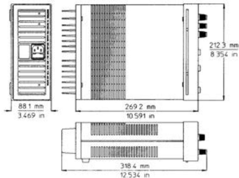
図 1: 外形図
