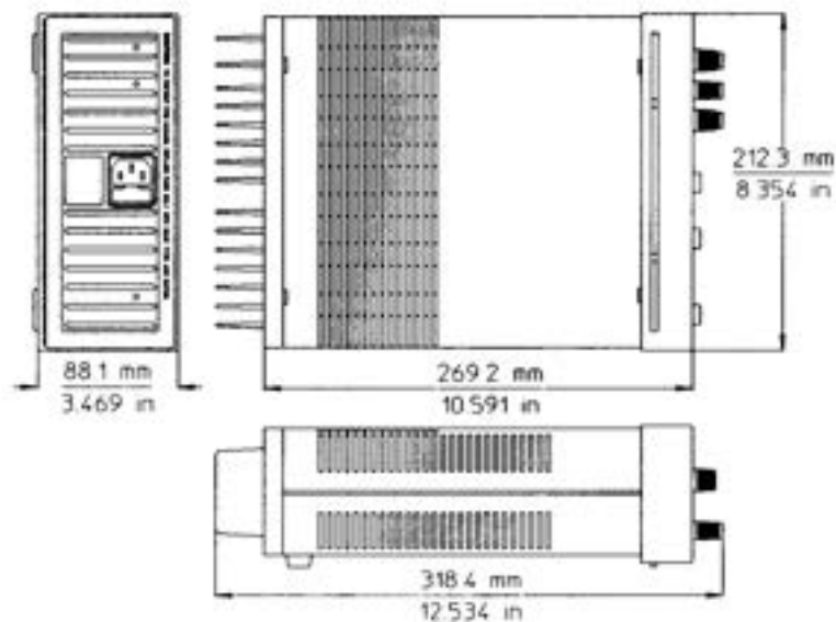
Figura 1: DIAGRAMA DESCRIPTIVO
